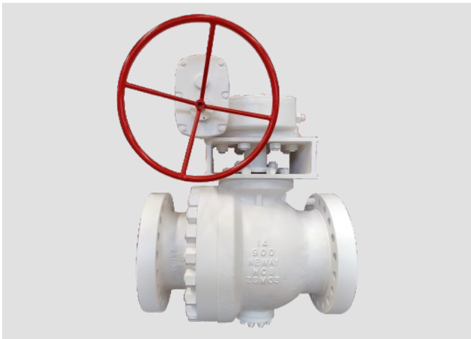
14"900LBC型球阀
