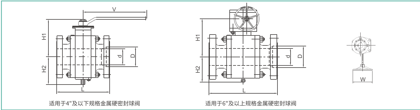
Class 900 全通径
