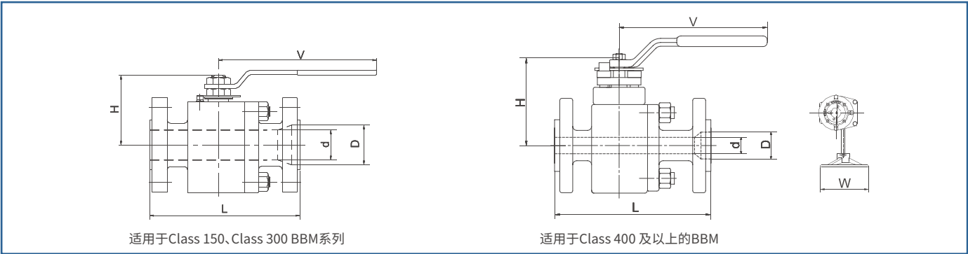
Class 600 全通径
