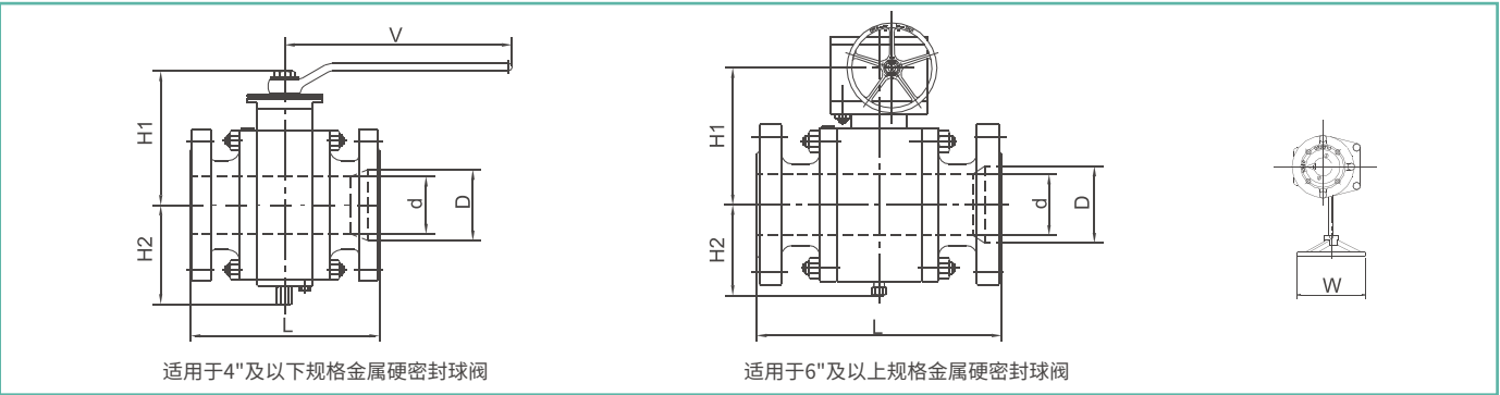
Class 300 全通径
