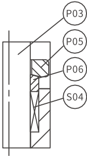
阀杆密封
