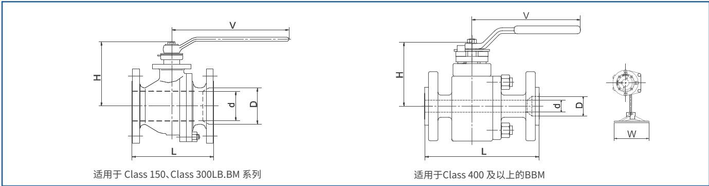
Class 300 缩径
